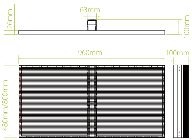
XRW8 Size
