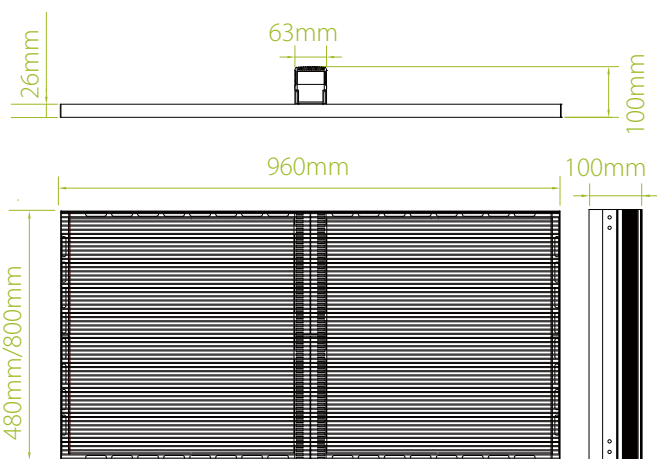
XRW10 Size
