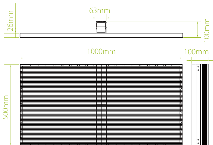
XRW3 Size
